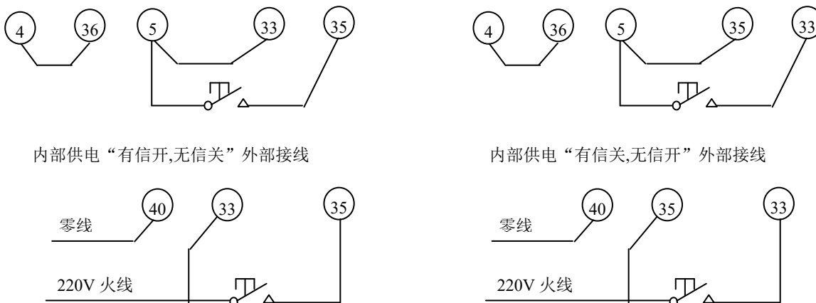
内部供电“有信开,无信关”外部接线
