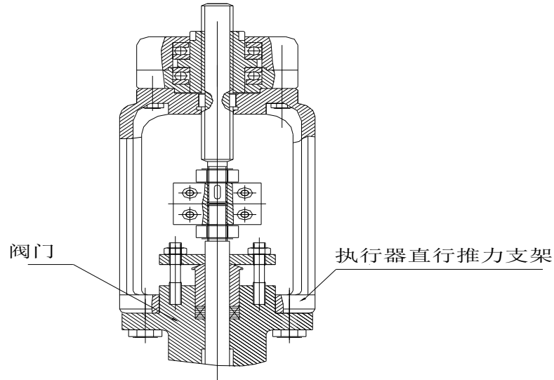
图 6-2 RQIII003~RQIII060、RQMIII03~RQMIII54 型执行机构丝杠与阀门连接形式示意图
