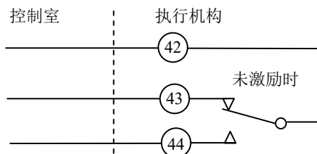
图 15-11 监视继电器接线图 (未激励时 42 与 43 为常闭端)
