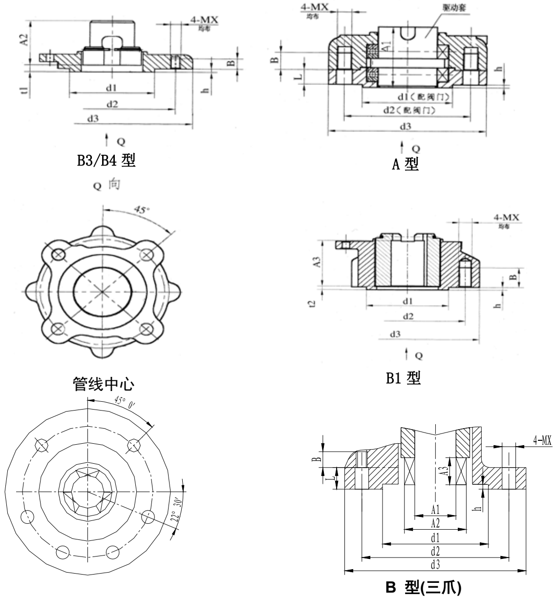
图 6-8 电动执行机构输出端与阀门连接法兰
