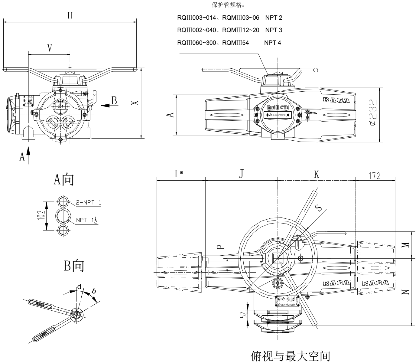
图 6-4 RQIII003~ RQIII100、RQMIII型执行机构安装尺寸图
