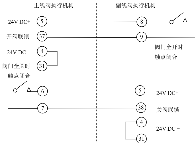
图 15-12 联锁功能应用实例
